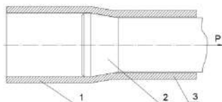
Схема процесса раздачи длинномерной трубы 1 – готовая труба, 2 – инструмент, 3 – заготовка.
